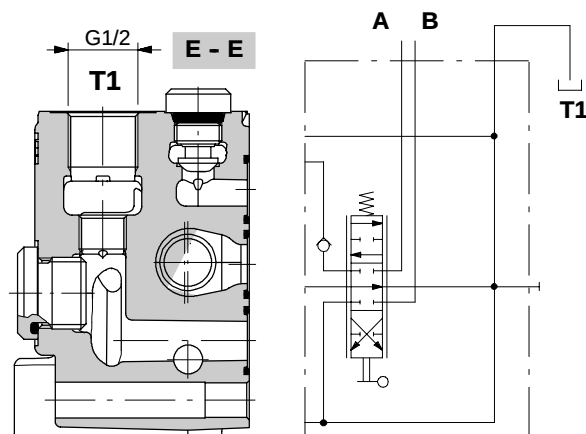
Description example: RQ-101-8L-TA
